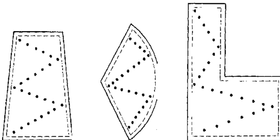
Рисунок 1 - W-образное распределение мест проведения измерений
