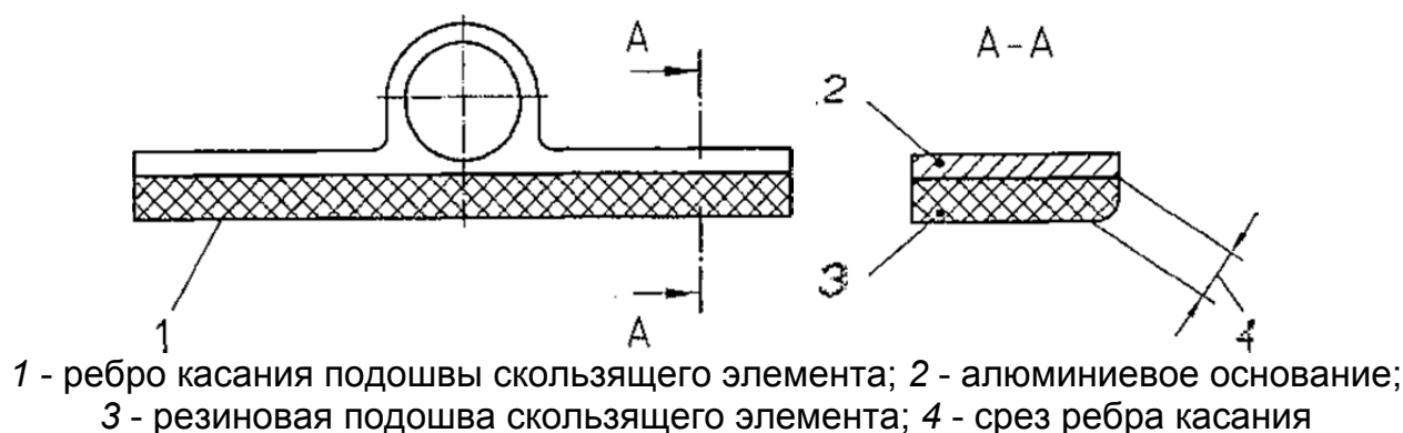
Рисунок 8 - Скользящий элемент
