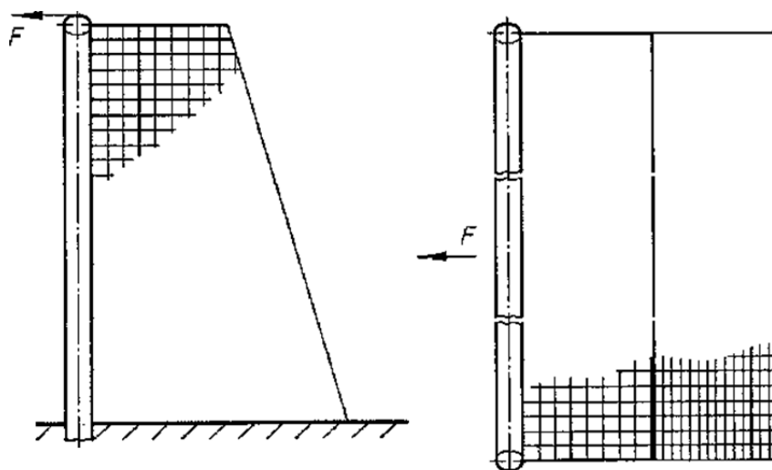
Рисунок 11 - Проверка стабильности ворот для футбола
