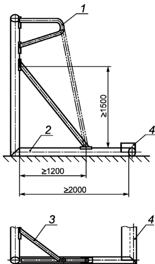
1 — консоль; 2 — наземная часть рамы; 3 — угловой кронштейн; 4 — противовес
